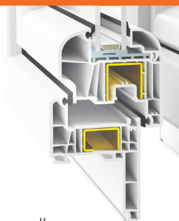
Profil trzyuszczelkowy
